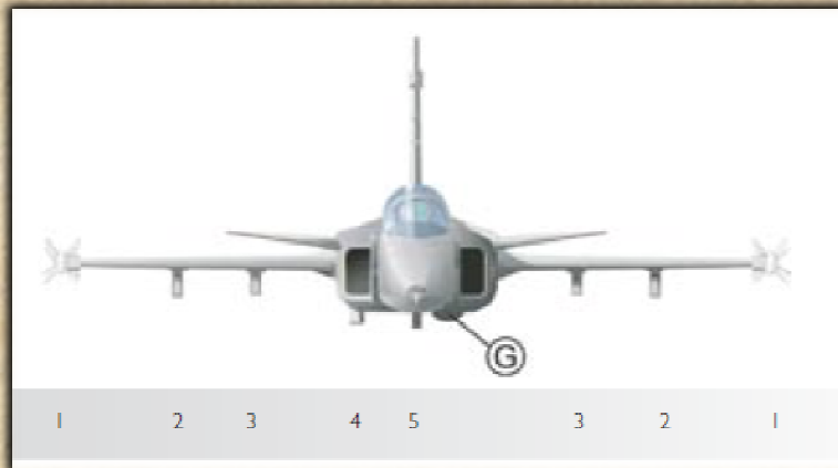
A JAS-39 C/D gépek felfüggesztési pontjai.
